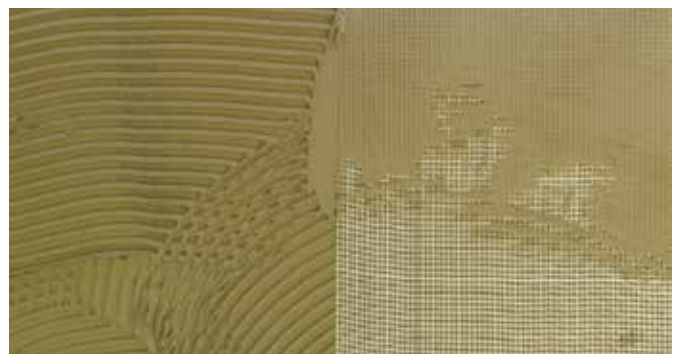
Üvegszövet háló beágyazása a felhordott rendszerragasztó rétegbe
